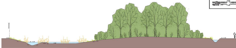
Principeprofiel riolevoer noordzijde, E-E'
